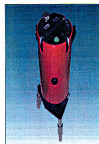
Roto-Sure 500 測距輪 1.直徑：160mm 2.精度：99.90%(25mm/30m) 3.重量：1.10 kg
