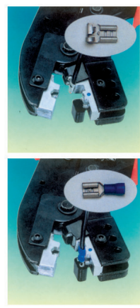
旗型端子、絕緣端子兩用
