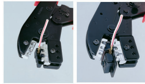
連續端子壓著鉗
